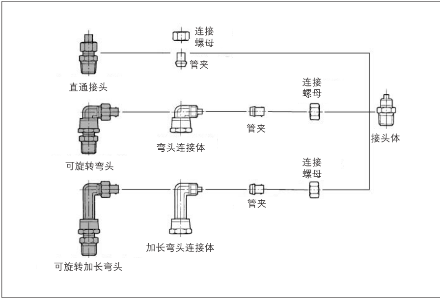
弯头连接体:KFV
